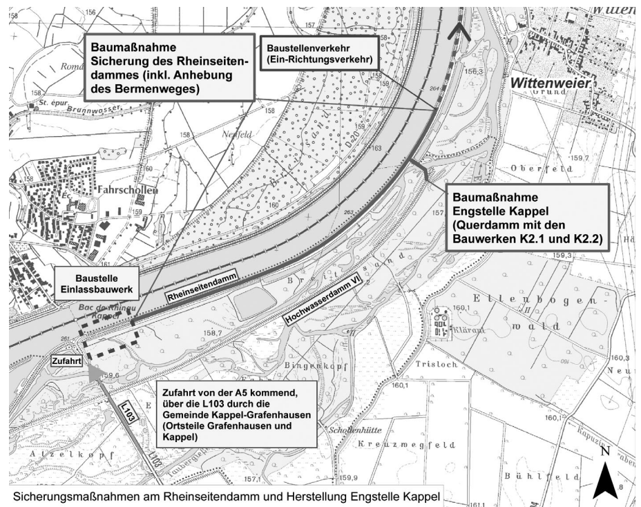
Sicherungsmaßnahmen am Rheinseitendamm und Herstellung Engstelle Kappel
